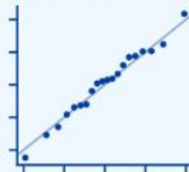
Quantile-Quantile Plot
